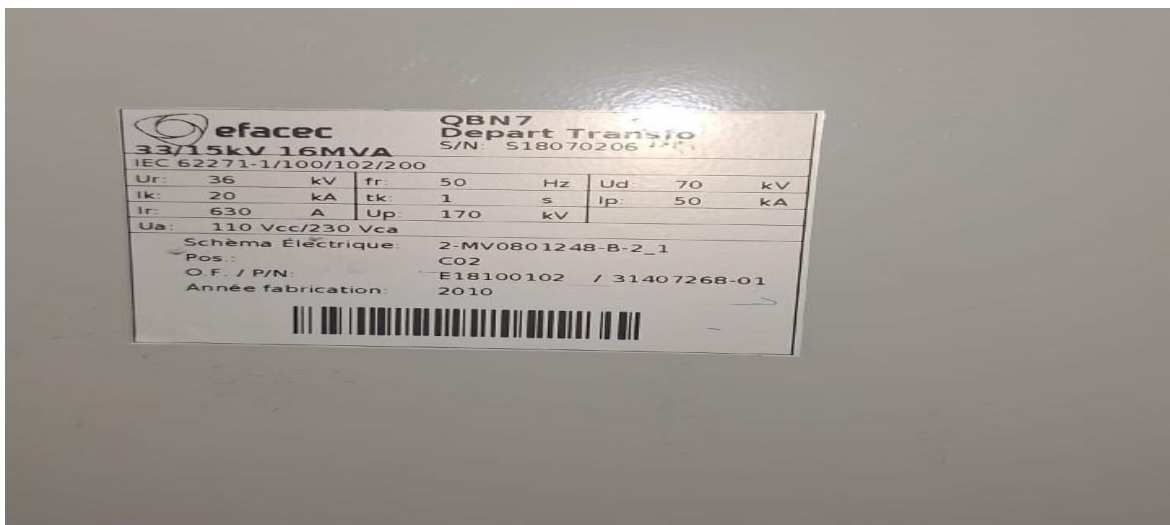
Img3 : Plaque signalétique de la cellule transfo 33kV
