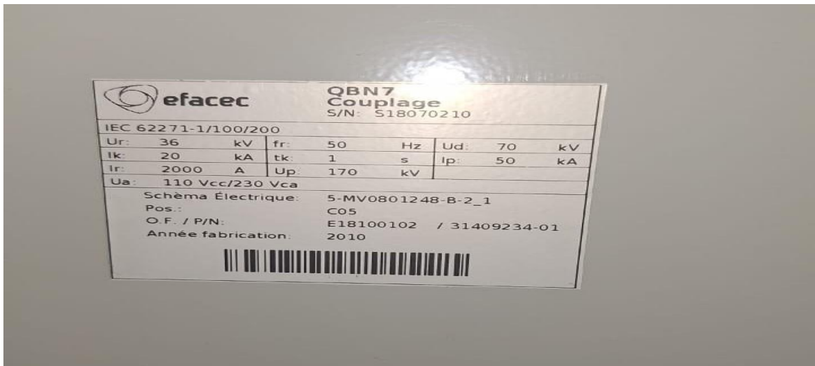
Img2: Plaque signalétique de la cellule couplage 33kV
