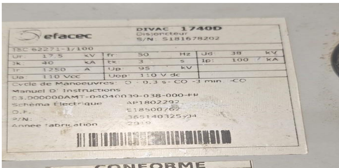
Img4 : Plaque signalétique du disjoncteur 15kV
