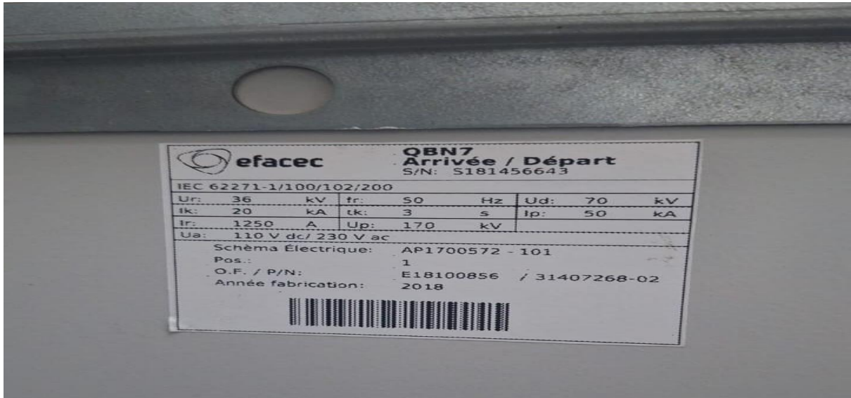
Img1 : Plaque signalétique de la cellule Départ 33kV
